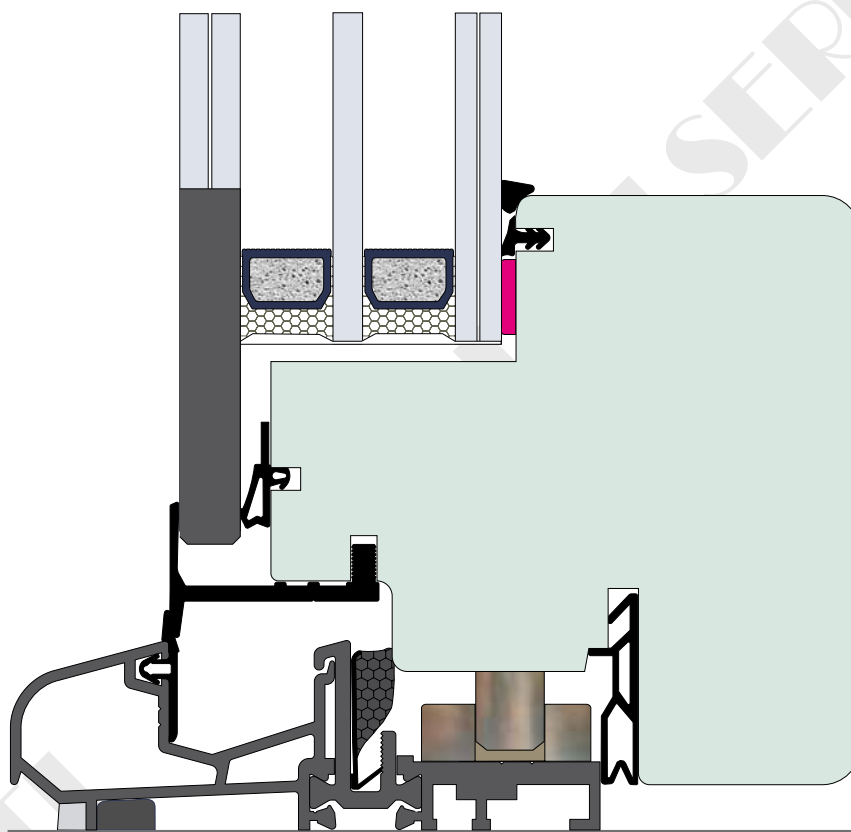
Particolare trasverso inferiore finestra e portafinestra
