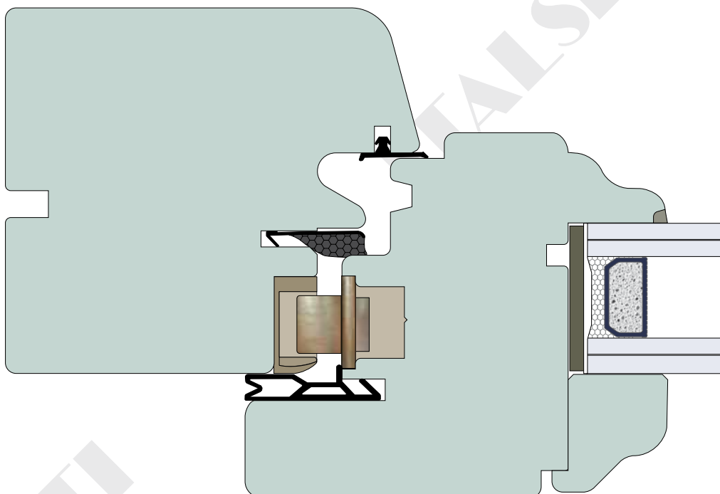
Particolare nodo laterale
