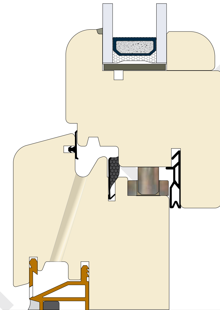
Particolare trasverso inferiore finestra
