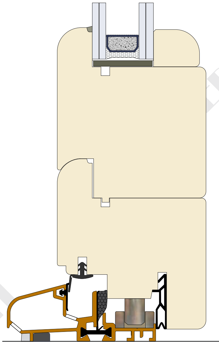
Particolare trasverso inferiore portafinestra
