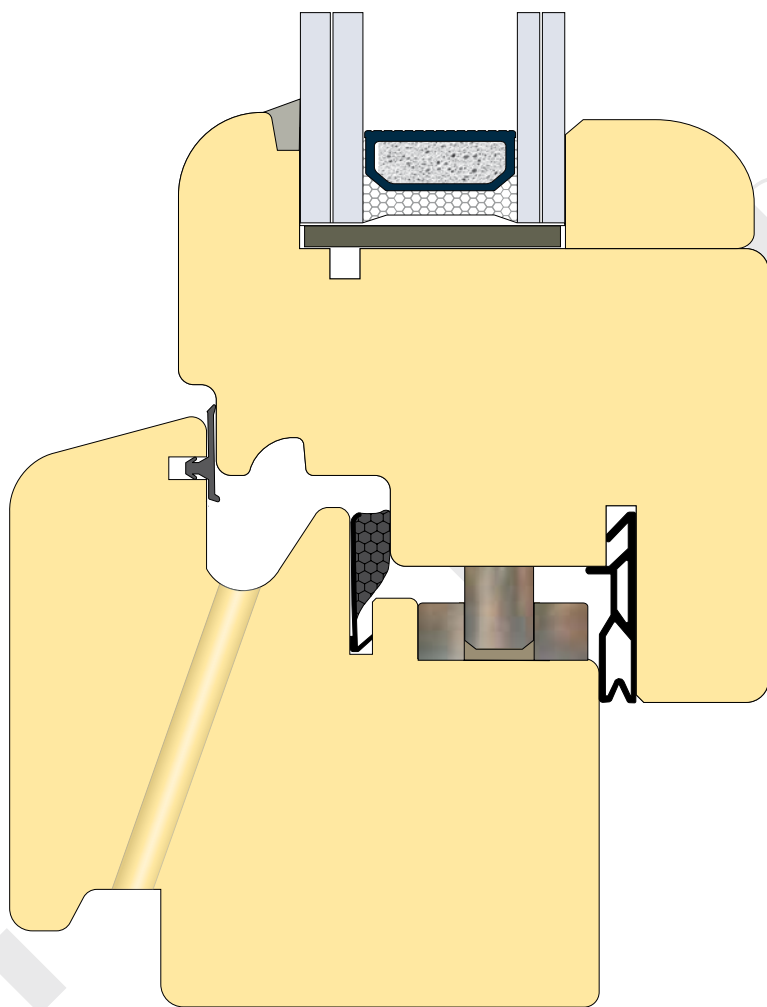
Particolare soglia finestra con traverso inferiore in legno (a richiesta)
