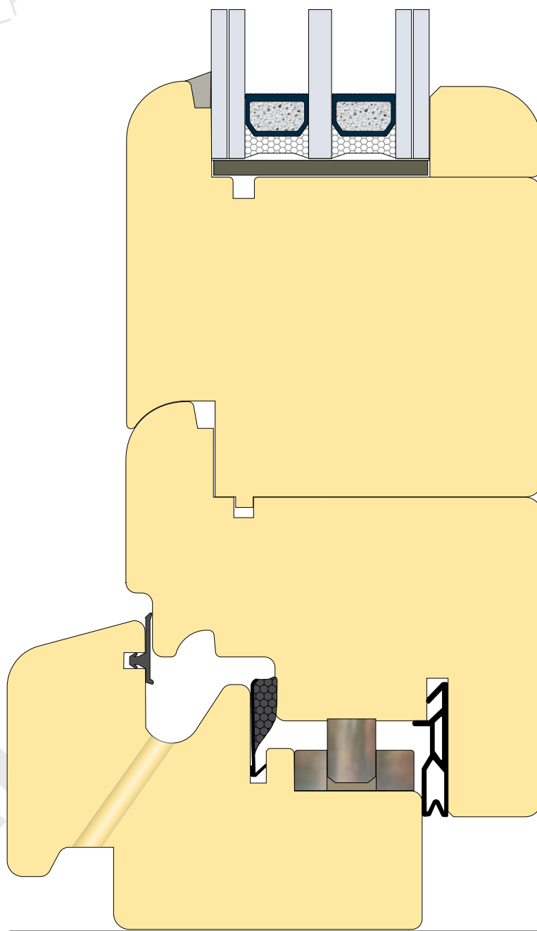
Particolare soglia porta finestra con traverso inferiore in legno (a richiesta)
