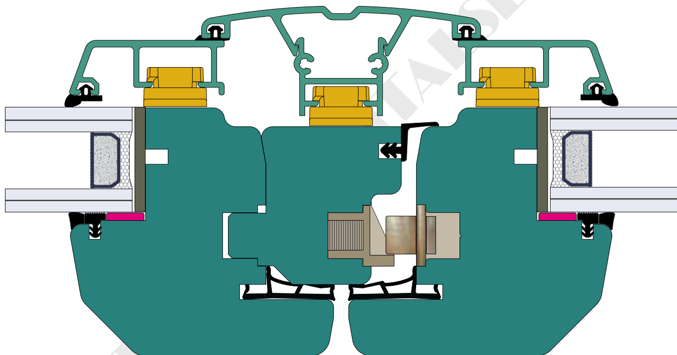
Particolare nodo centrale
