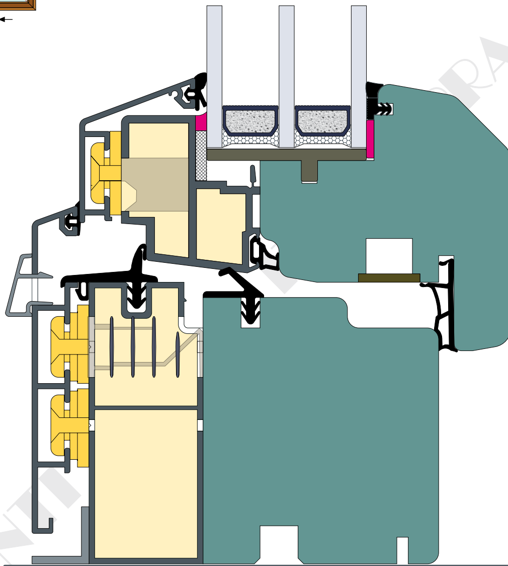
Particolare trasverso inferiore finestra (std)
