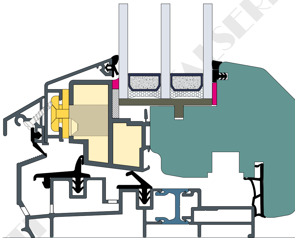
Particolare trasverso inferiore portafinestra (std)
