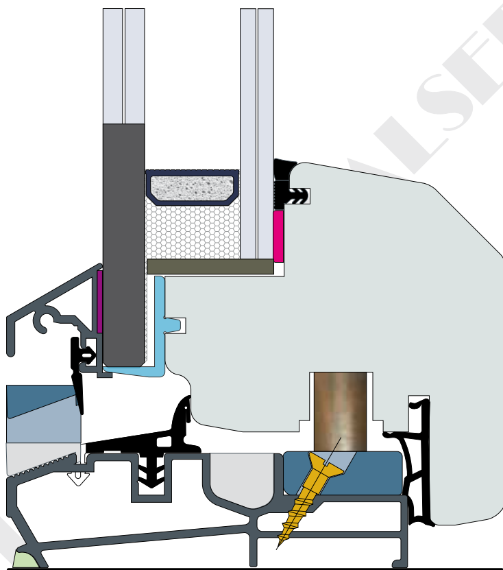
Particolare trasverso inferiore finestra (std)
