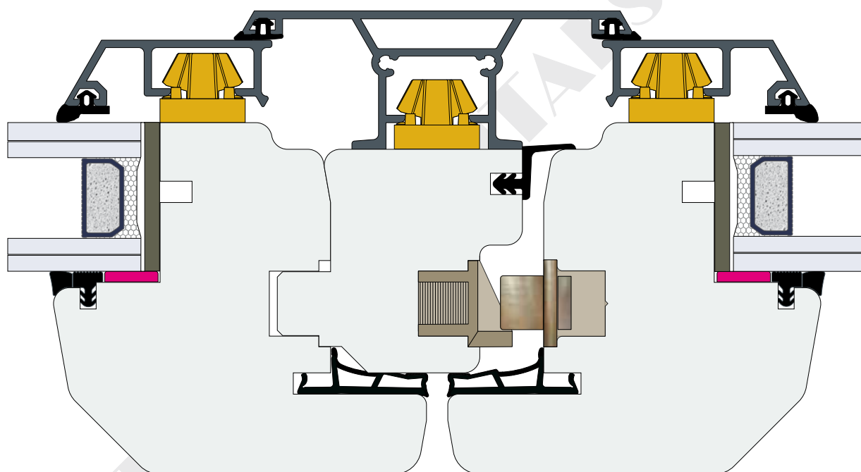
Particolare nodo centrale
