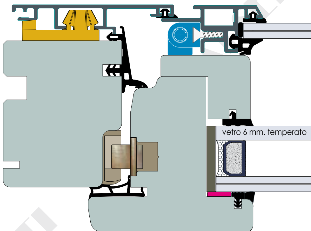
Particolare nodo laterale
