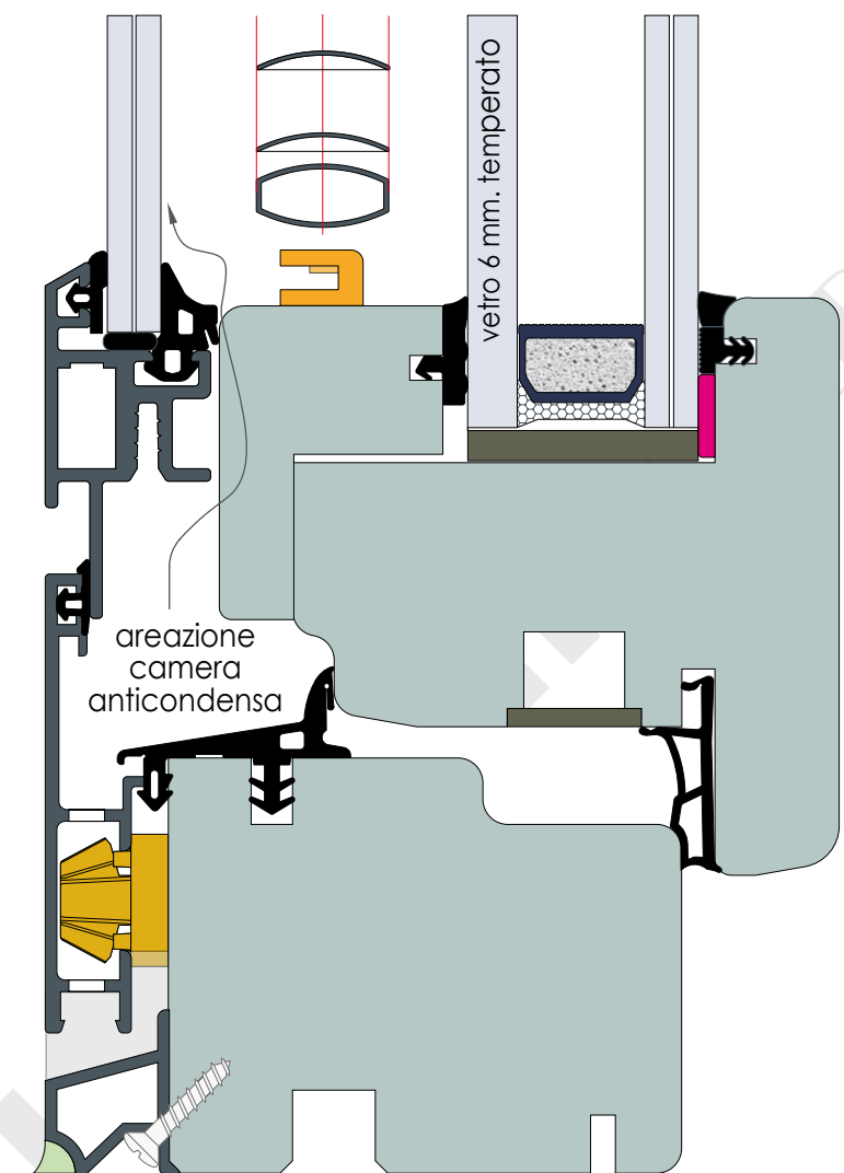
Particolare traverso inferiore finestra (std)
