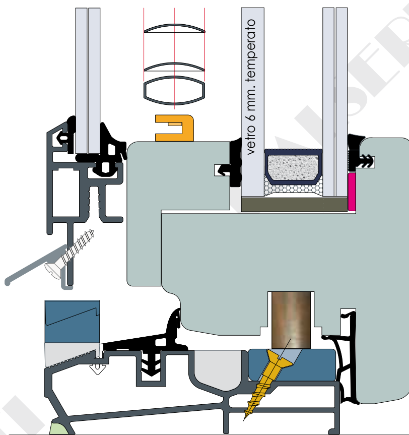
Particolare trasverso inferiore portafinestra (std)
